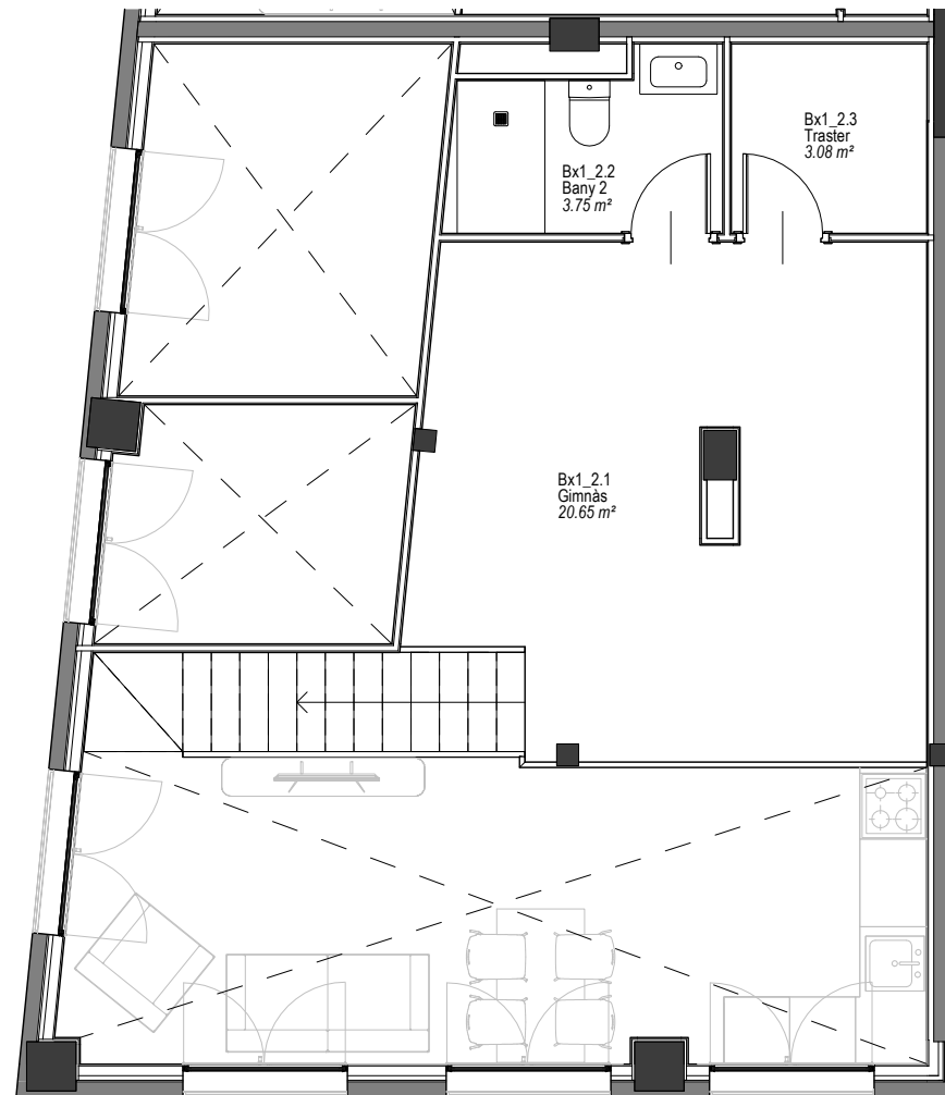
HABITATGE B1 Planta altell
