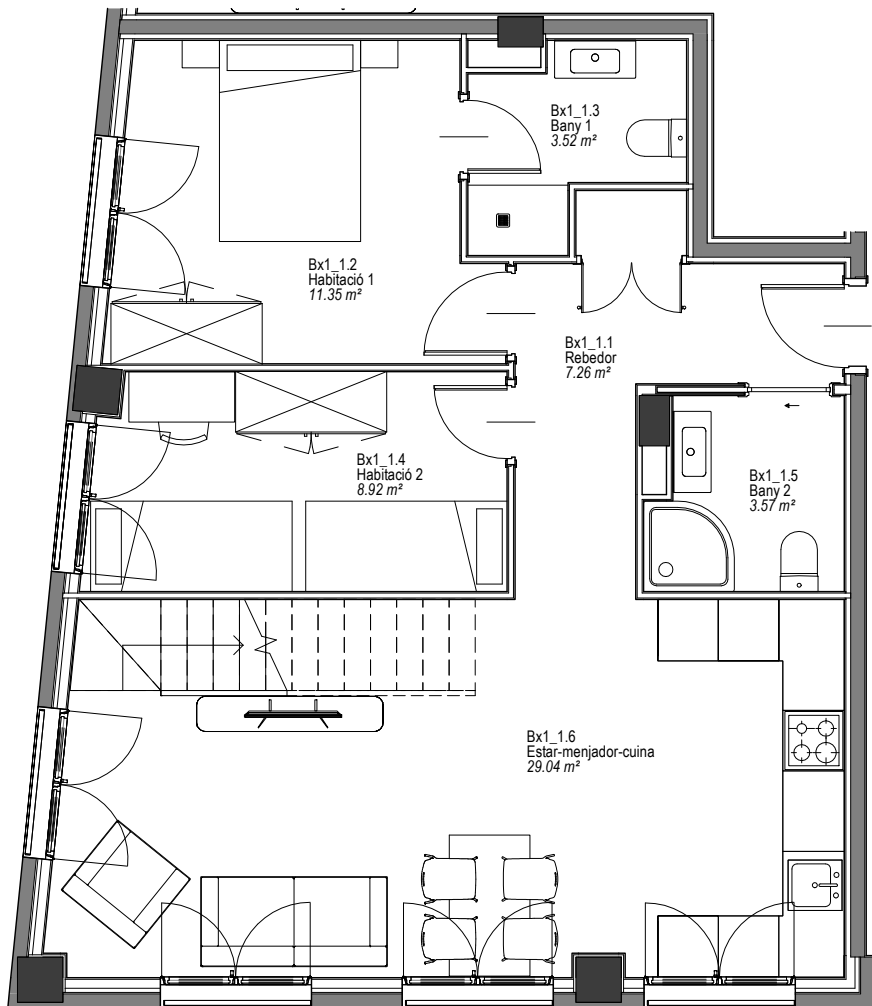
HABITATGE B1 Planta baixa
